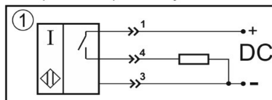
Цоколевка разъема
