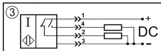
Переключающий контакт
