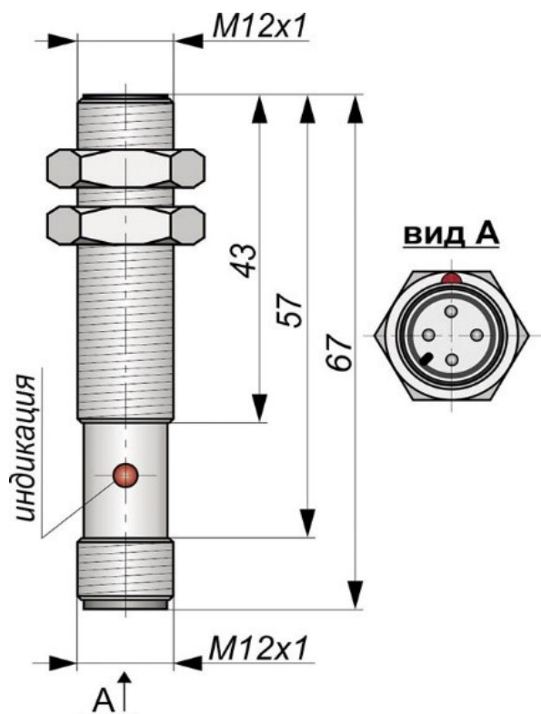
Габаритный чертеж
