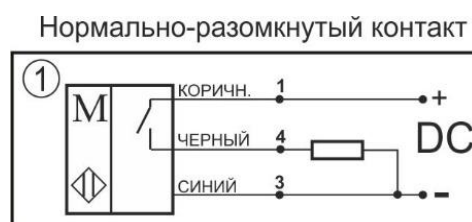
Схема соединения
