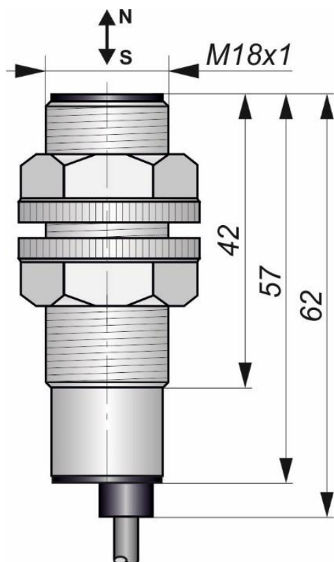
Габаритный чертеж
