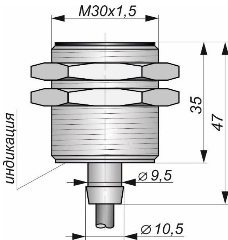
Габаритный чертеж
