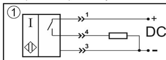
Цоколевка разъема
