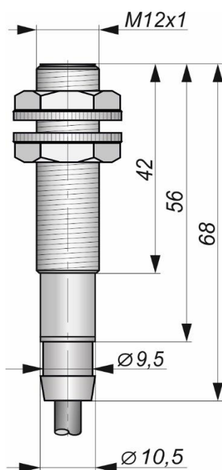
Габаритный чертеж
