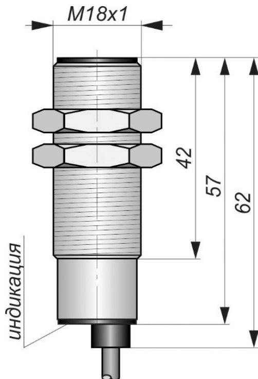
Габаритный чертеж
