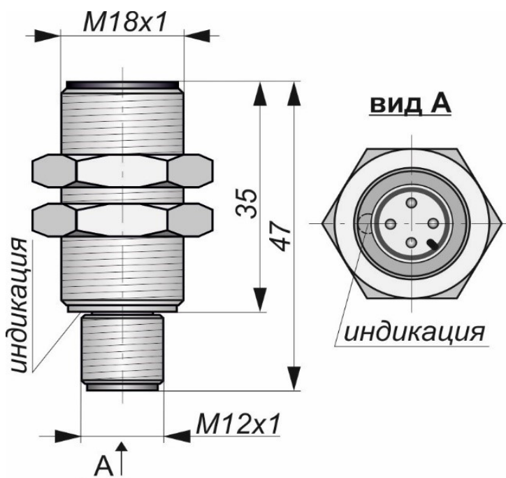
Габаритный чертеж
