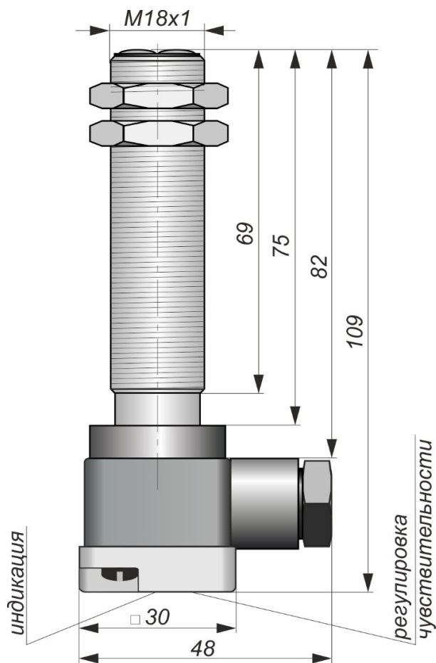
Габаритный чертеж
