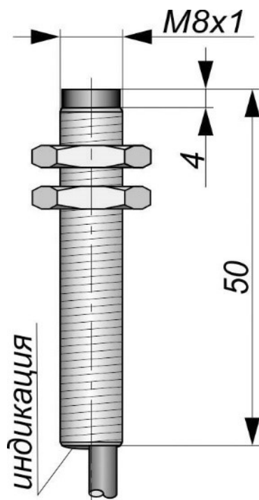
Габаритный чертеж
