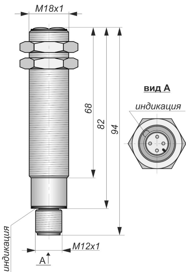
Габаритный чертеж
