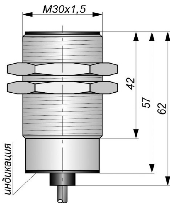
Габаритный чертеж
