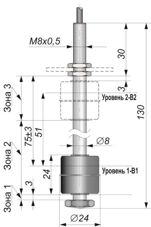
Габаритный чертеж
