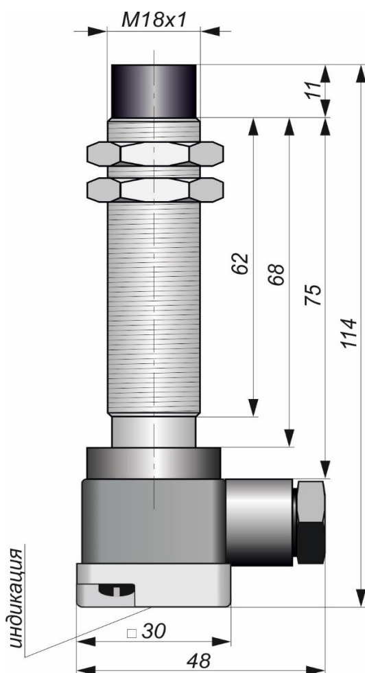
Габаритный чертеж
