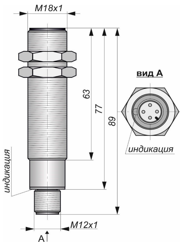
Габаритный чертеж
