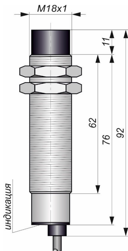
Габаритный чертеж
