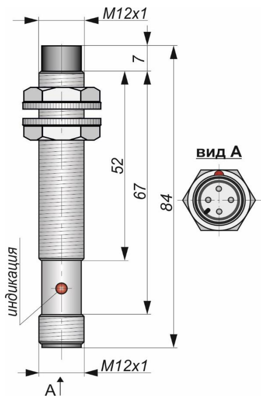
Габаритный чертеж
