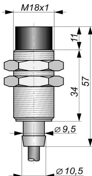
Габаритный чертеж
