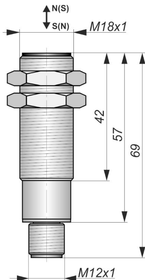
Габаритный чертеж
