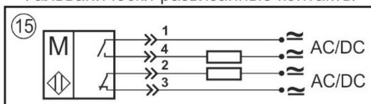
Гальванически-развязанные контакты
