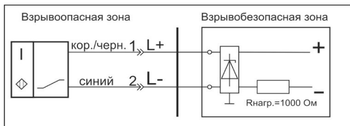
Схема соединения
