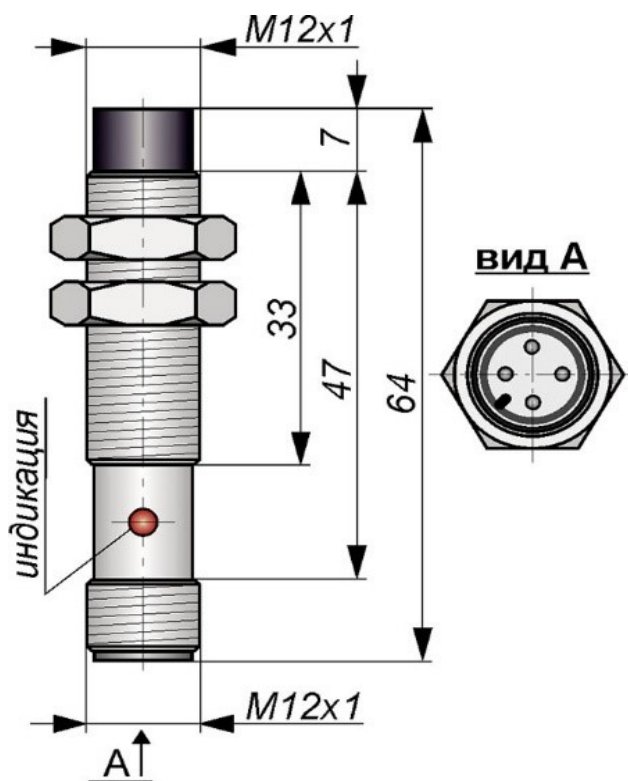
Габаритный чертеж
