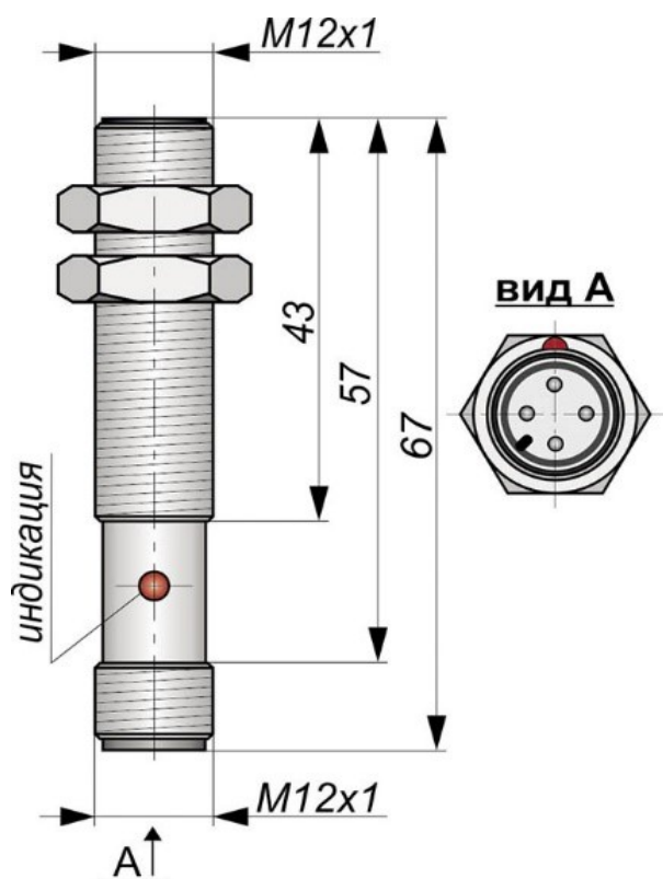
Габаритный чертеж
