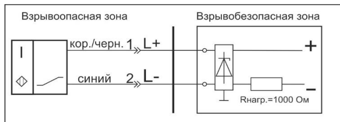
Схема соединения
