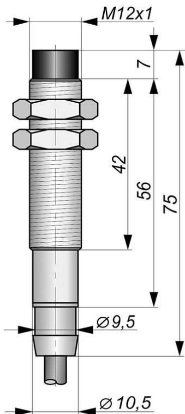
Габаритный чертеж
