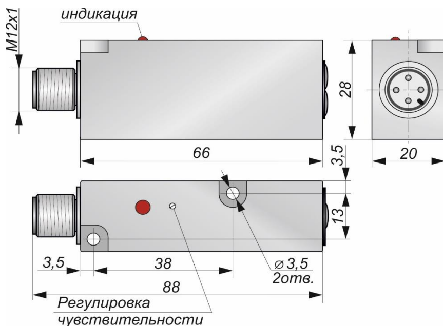
Габаритный чертеж
