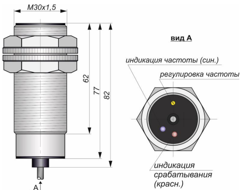
Габаритный чертеж
