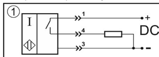
Нормально-разомкнутый контакт
