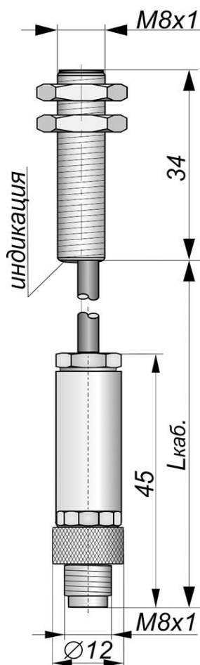
Габаритный чертеж
