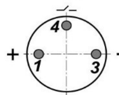
Цоколевка разъема
