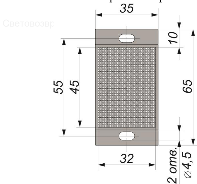
Габаритный чертеж
