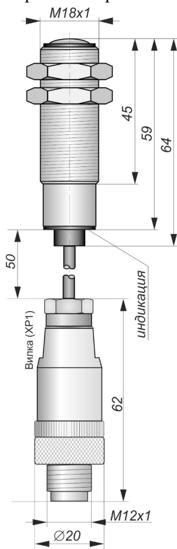
Габаритный чертеж
