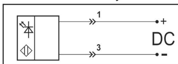
Цоколевка разъема
