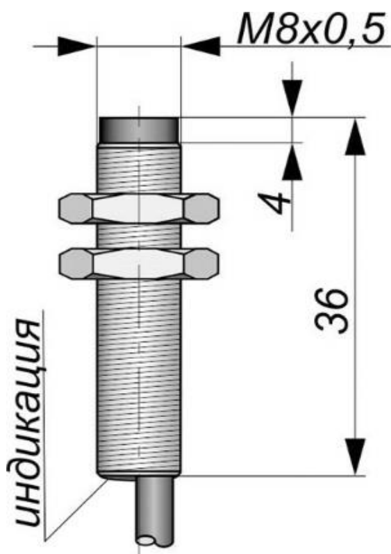
Габаритный чертеж
