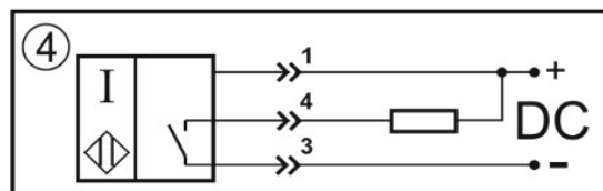
Нормально-разомкнутый контакт
