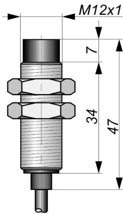
Габаритный чертеж
