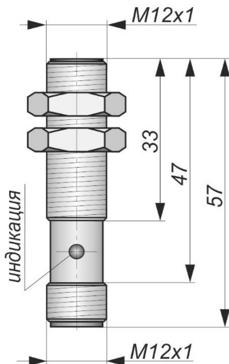
Габаритный чертеж
