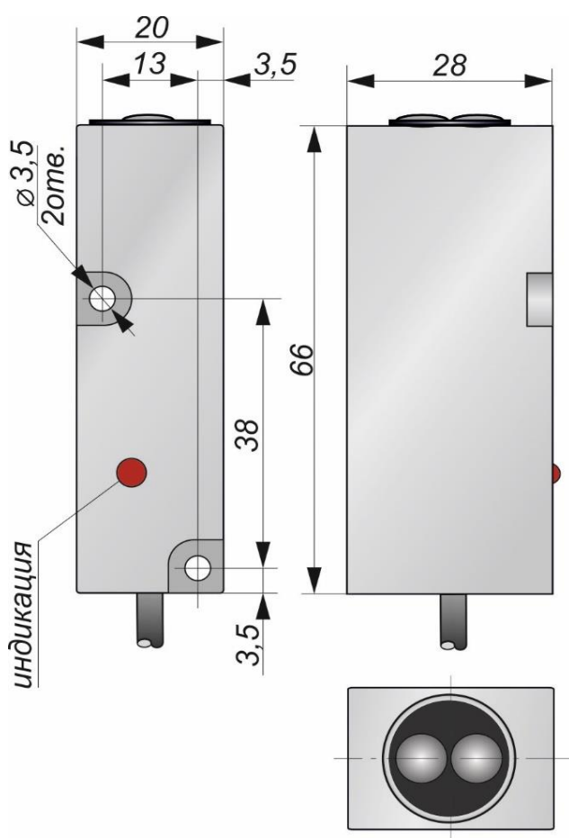
Габаритный чертеж
