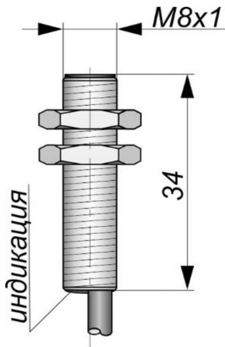
Габаритный чертеж
