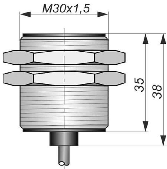
Габаритный чертеж
