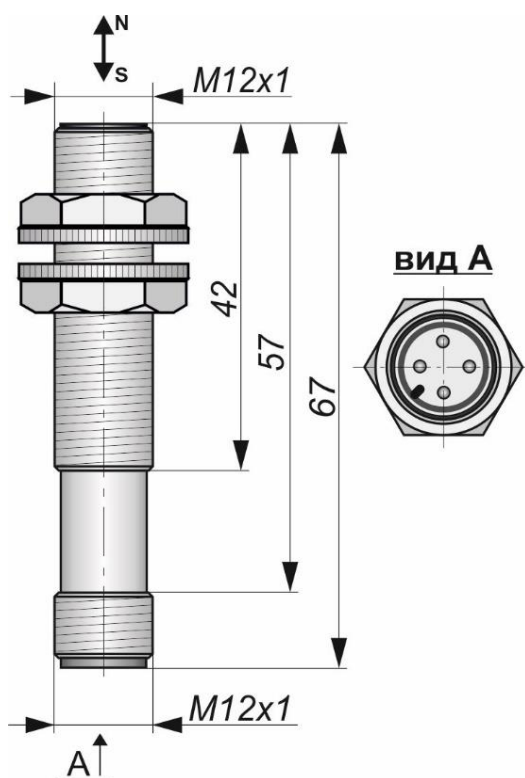
Габаритный чертеж
