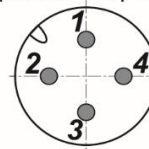
Цоколевка разъема
