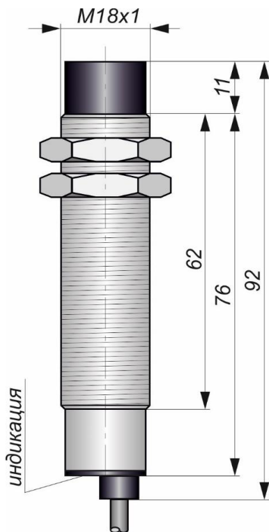
Габаритный чертеж
