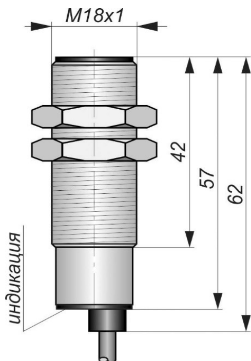
Габаритный чертеж
