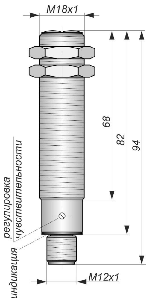
Габаритный чертеж
