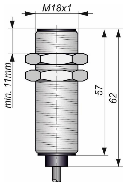
Габаритный чертеж
