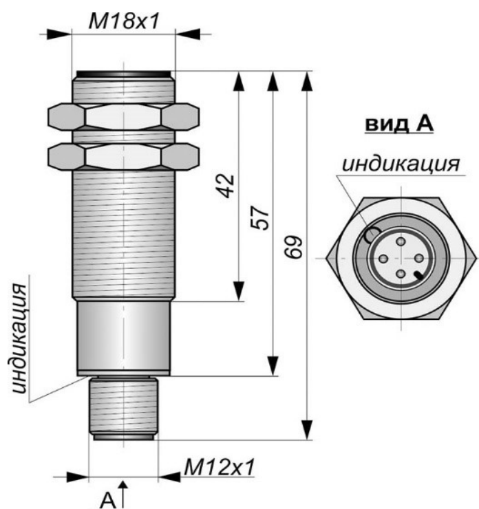
Габаритный чертеж
