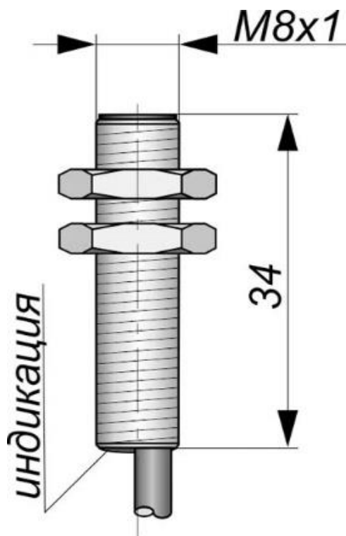
Габаритный чертеж
