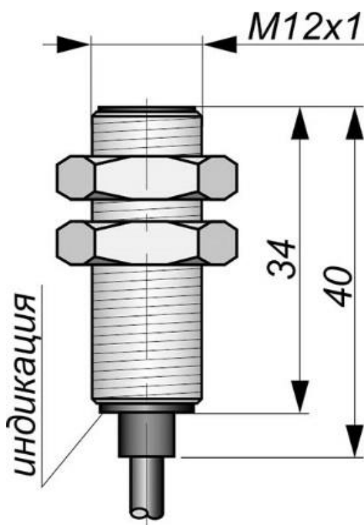
Габаритный чертеж
