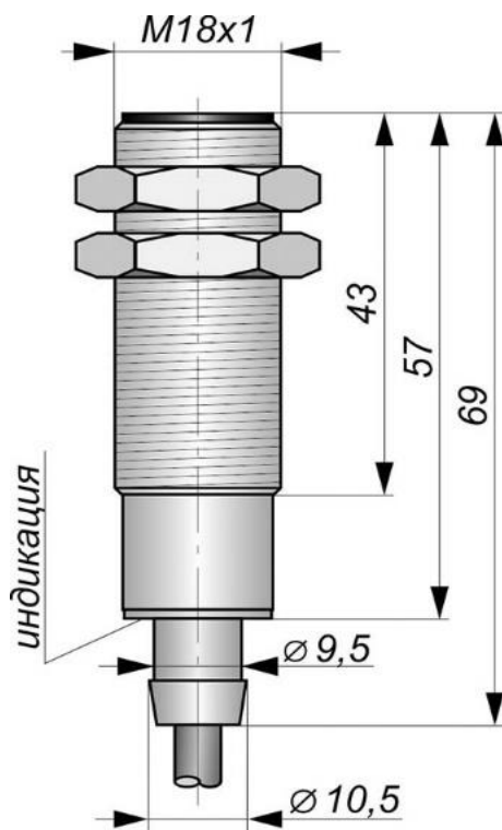
Габаритный чертеж
