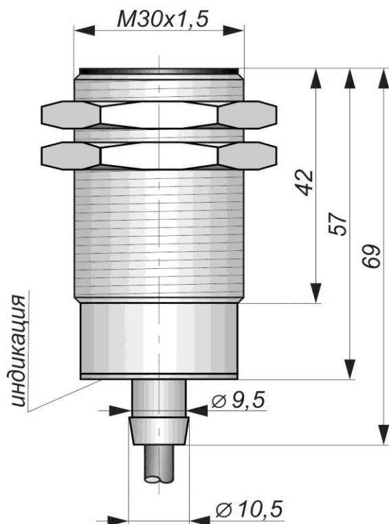
Габаритный чертеж
