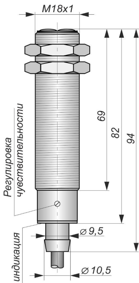
Габаритный чертеж
