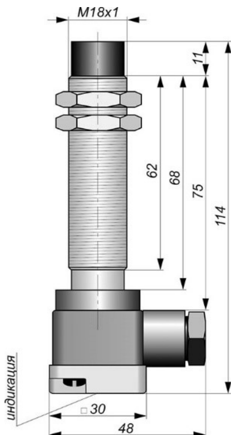
Габаритный чертеж
