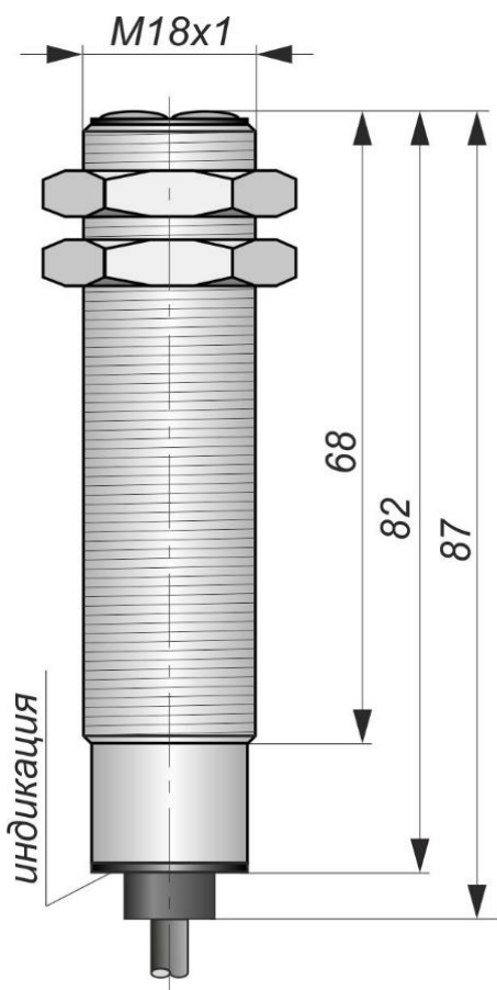
Габаритный чертеж
