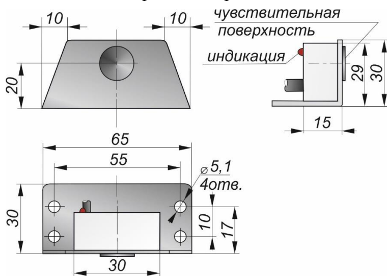
Габаритный чертеж
