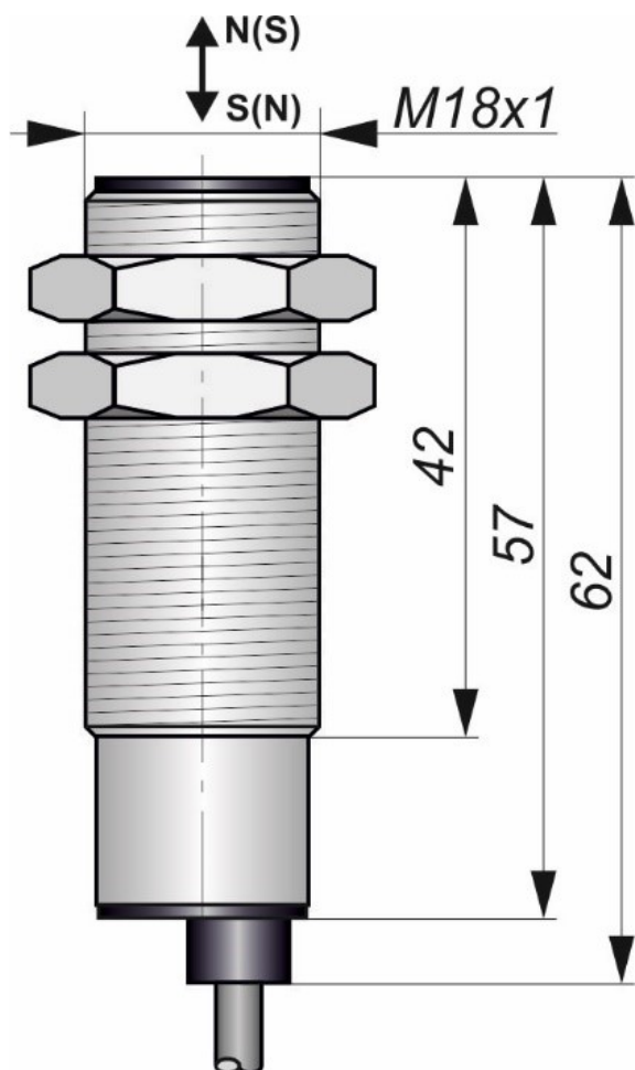
Габаритный чертеж
